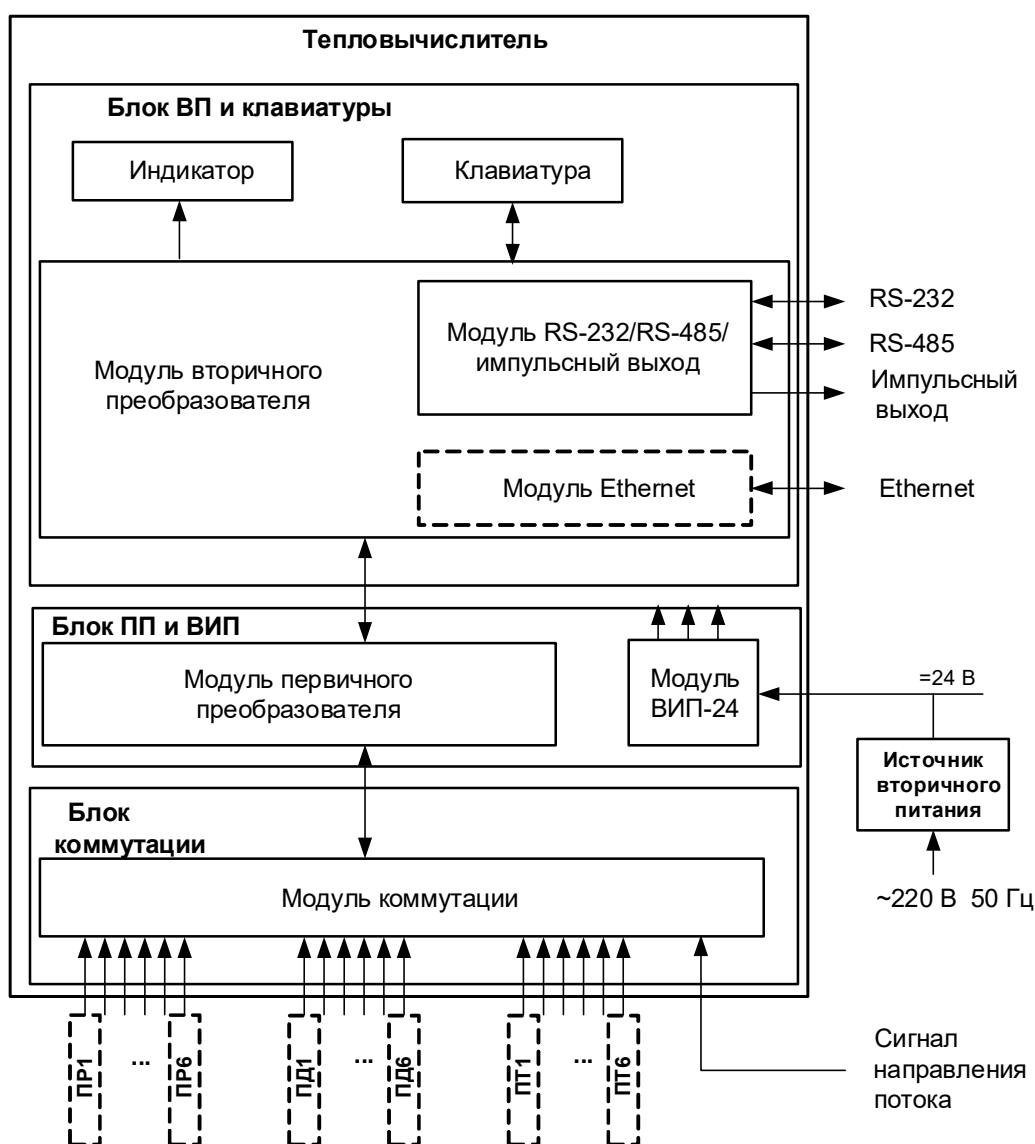
Рис.1. Структурная схема тепловычислителя.
