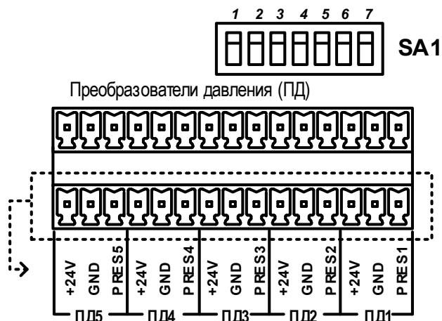
Рис.30. Обозначение коммутационных элементов подключения ПД.
